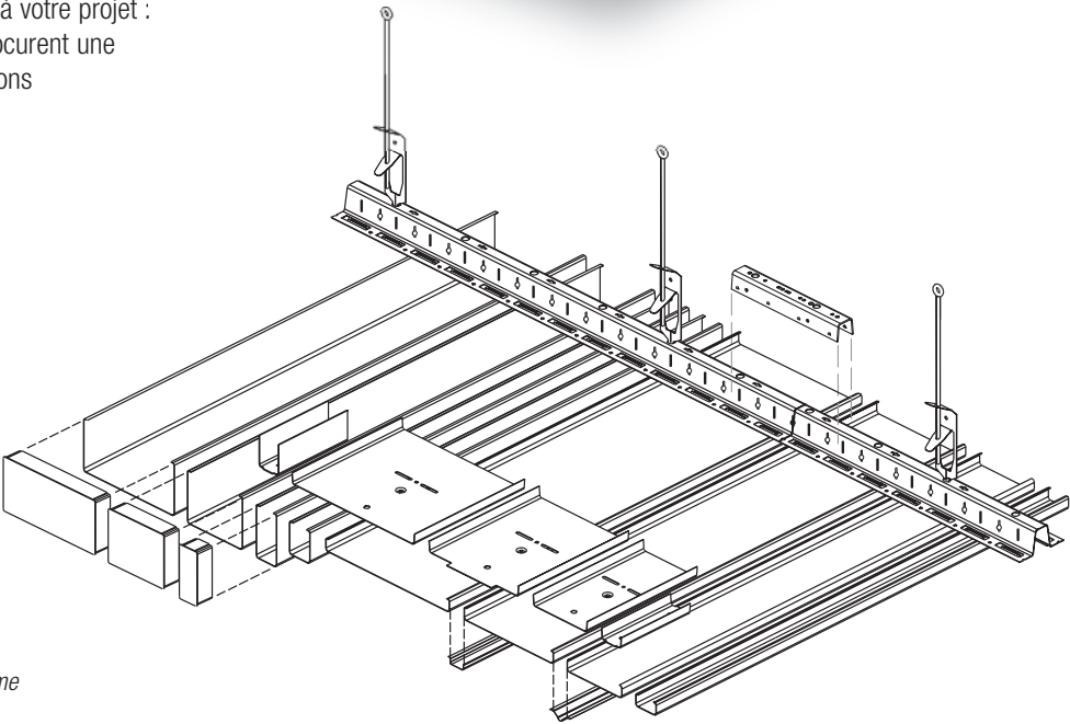
Lames de plafond 30BXD, 30BD et 130B
