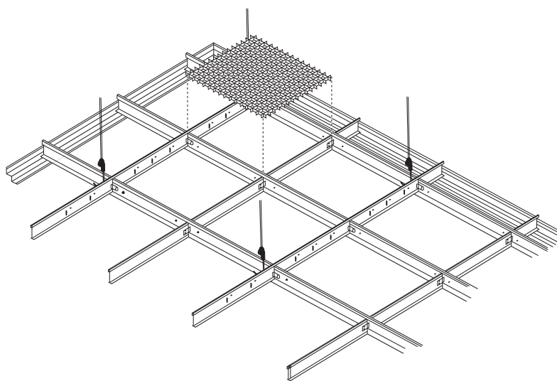
1. Lay-on (T24/T15)
