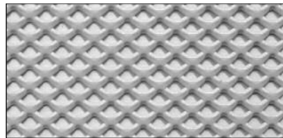
LS6 acier, surface d'ouverture 38%, épaisseur 1.7 mm
