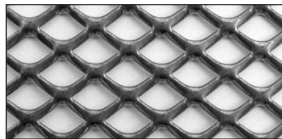
LS12 acier/aluminium, surface d'ouverture 72%, épaisseur 2.0 mm
