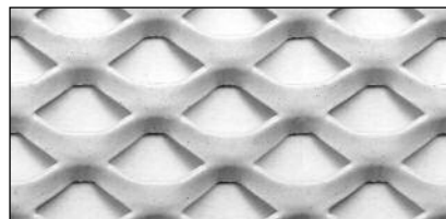
LS16 acier, surface d'ouverture 66 %, épaisseur 2.0 mm
