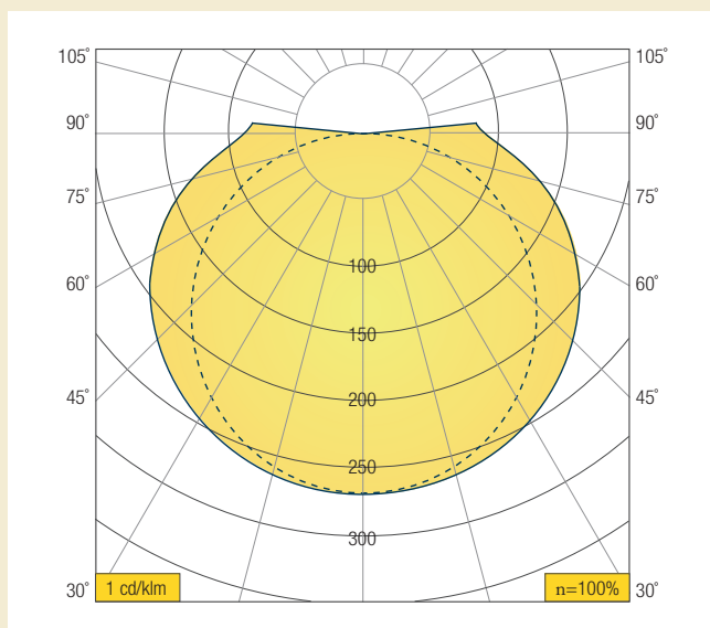
— C0,0 : mesurée par-dessous - - - - C90,0 : mesurée latéralement
