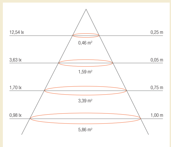
Mesure obtenue sur une Lightline Luxalon® de 960 mm en coloris blanc cassé
