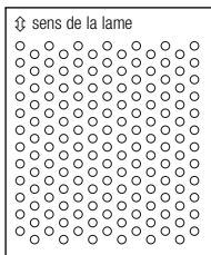
Ø 1 mm surface ouverte de 23% ⇄ 2 ⇄ 3,46
