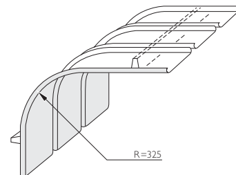
Cornière intérieure (rayon fixe)
