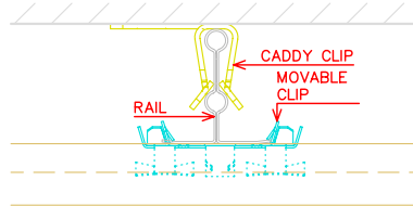
HORIZ. SECTIONS
